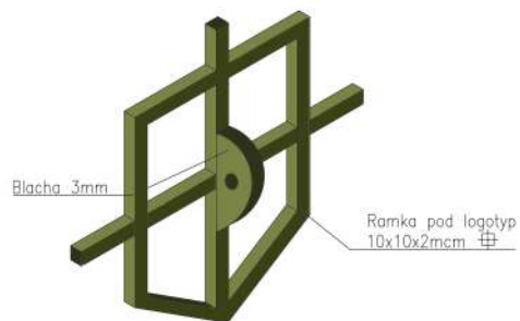
Detal łączenia
